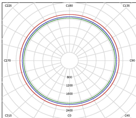
Oprawa: ELGIS OP-41 OP-41 Lampy: 1 x NAV 70W/E27
