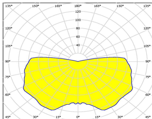
Oprawa: ELGIS OP-41 OP-41 Lampy: 1 x NAV 70W/E27
