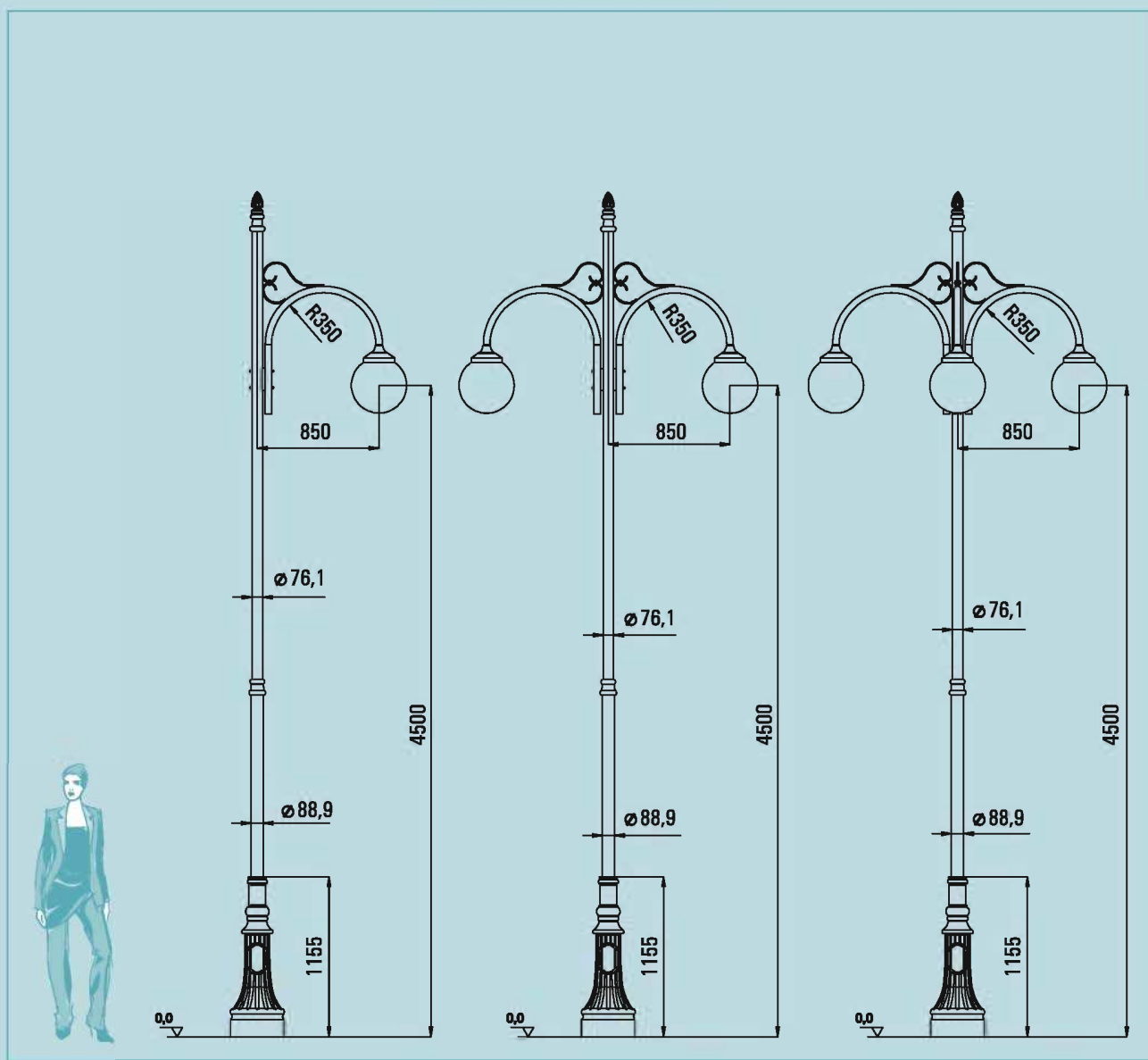
LP-6/4,5/1/OP
