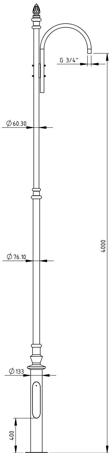
F80 wymiary
