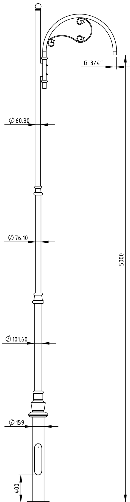
F80 wymiary
