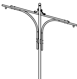
SPC-B-5/2/W6
