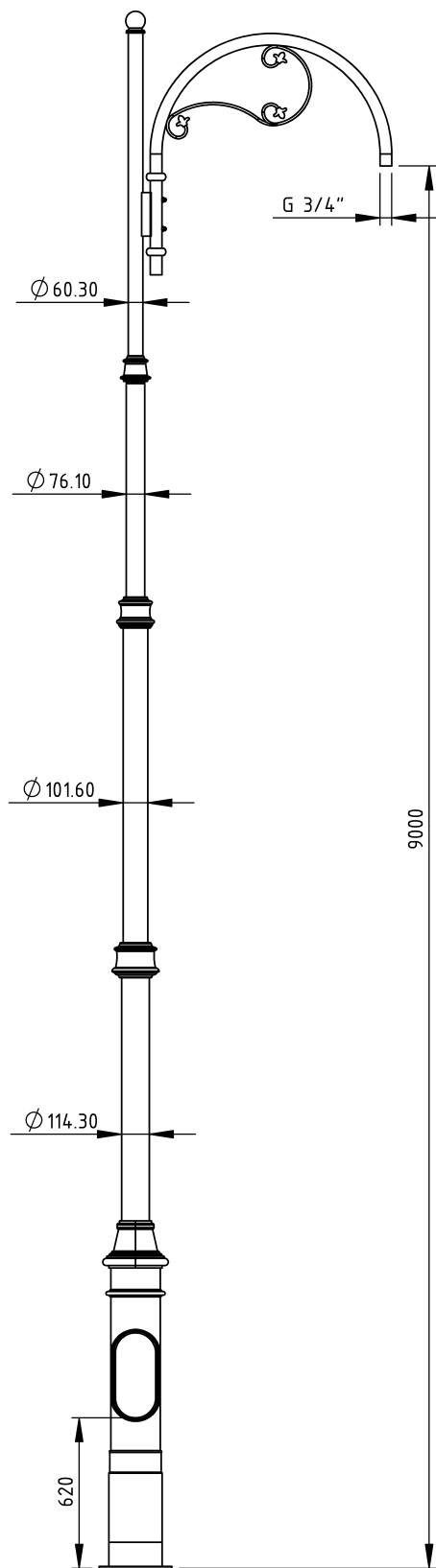
F150 wymiary
