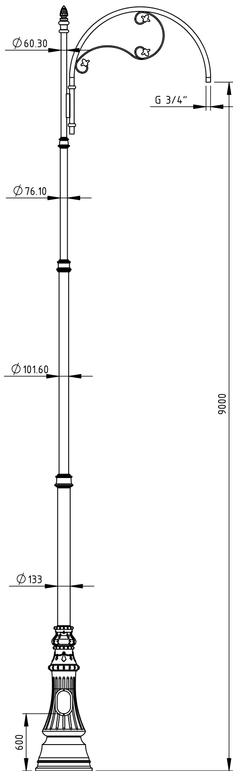
F150 wymiary
