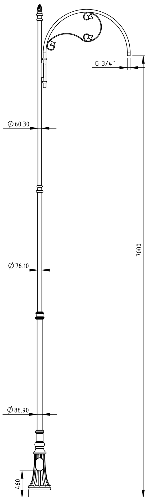
F150 wymiary
