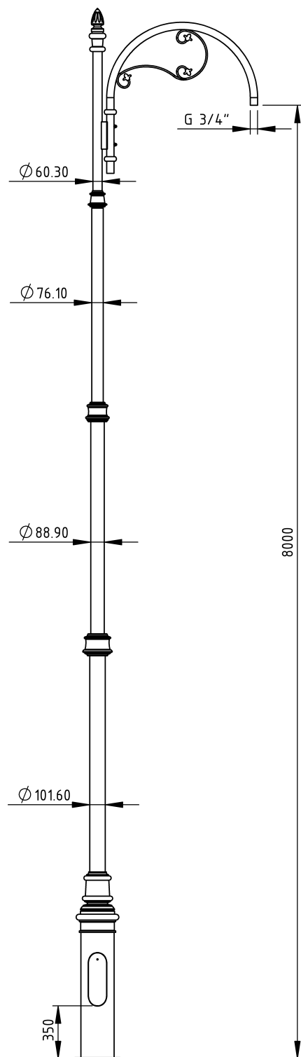
F150 wymiary
