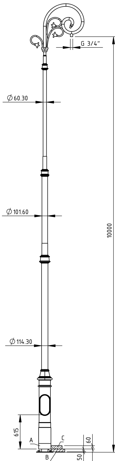
F150 wymiary
