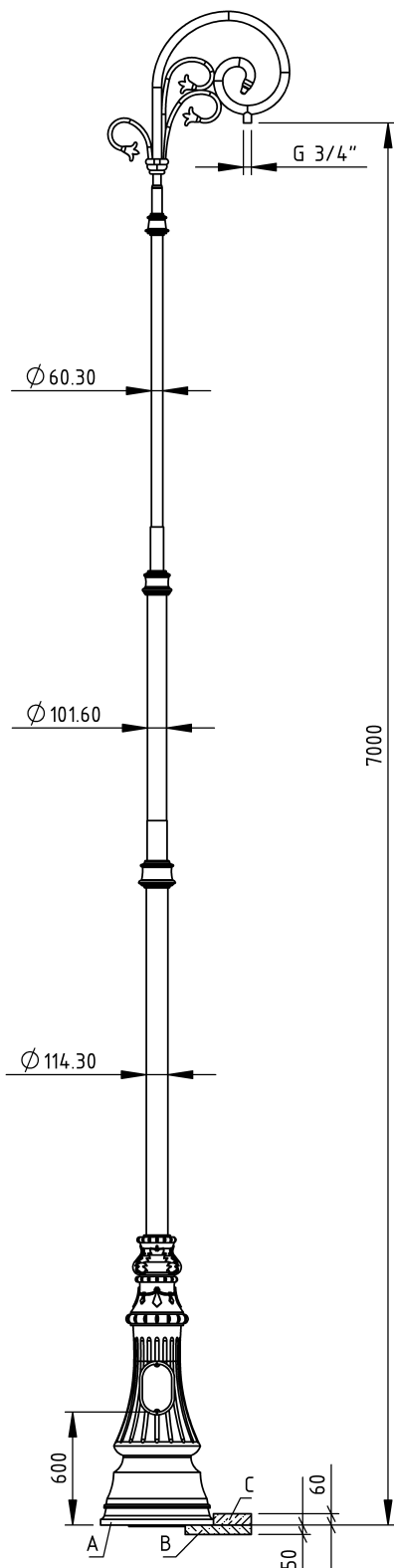
F150 wymiary
