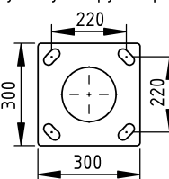
wymiary stopy słupa
