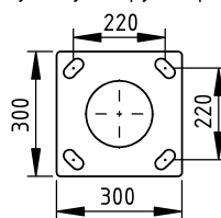
wymiary stopy stupa
