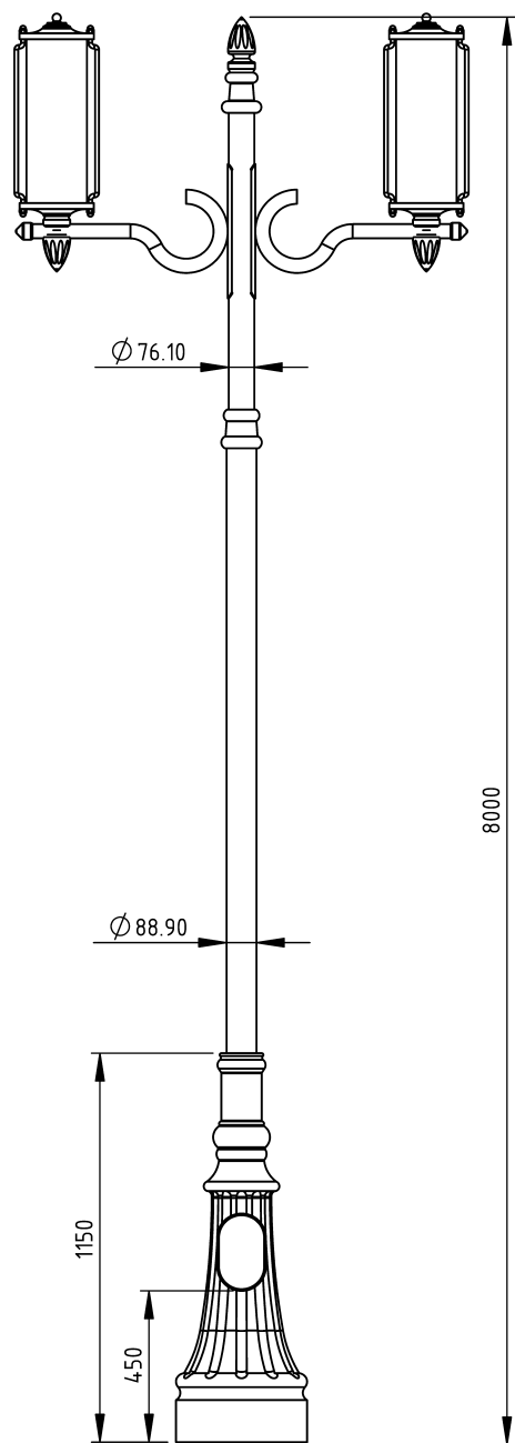
F150 wymiary
