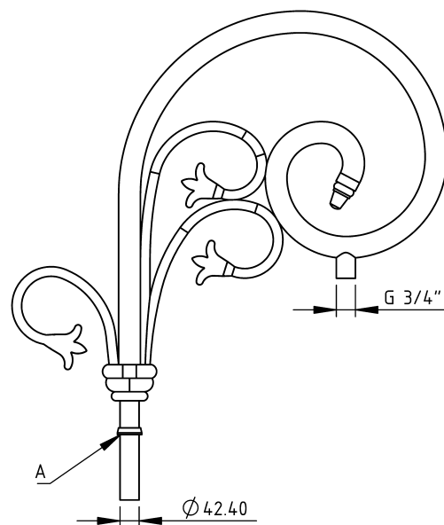
A - wysięgnik spawany na stałe do słupa
