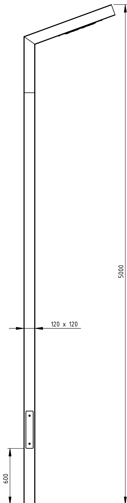
F80 wymiary
