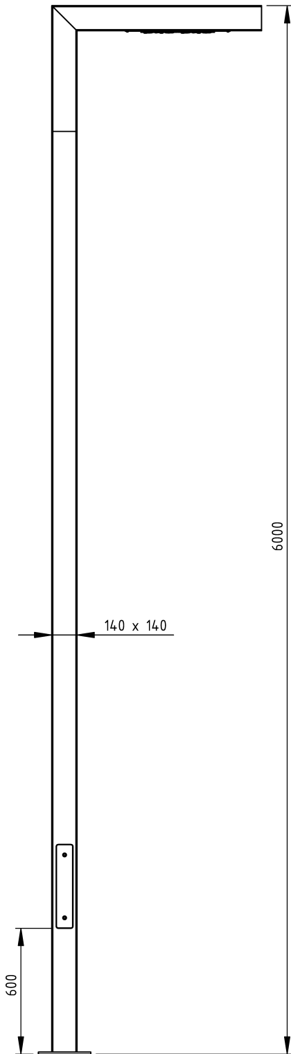
F100 wymiary
