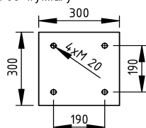
F80 wymiary
